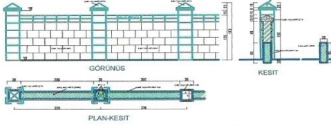
BAHÇE DUVARI DETAYI ( D1 )
